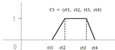
Рисунок 1. Трапециевидное число
